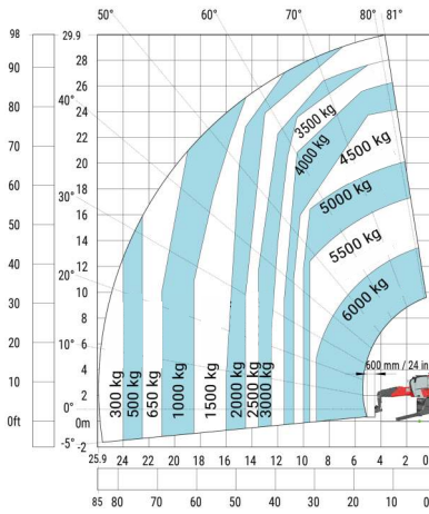
Makina ayaklar üzerinde vinçli jib ataşmanı ile
