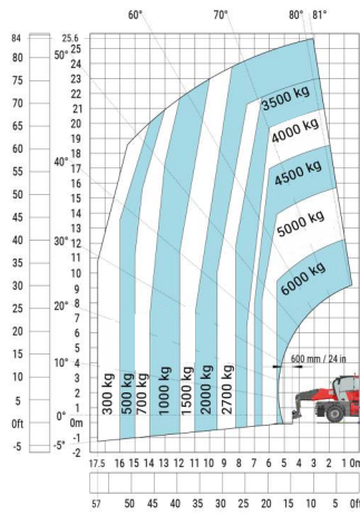
Makina ayaklar üzerinde vinçli jib ataşmanı ile
