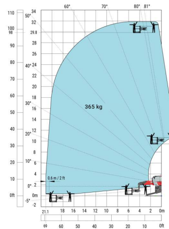
Makina ayaklar üzerinde 365 kg personel platformu ile
